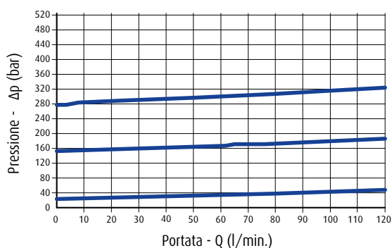
Molla Spring 20/280 Bar
